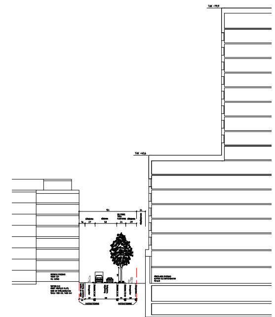
Sektion D-D Ernst Fontells Plats, norr om Smålandsgatan Skala 1:1000 (A4)
