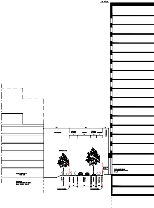
Sektion E-E Ernst Fontells Plats, mot Skånegatan Skala 1:1000 (A4)
