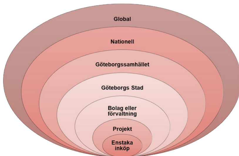
Figur 3 Schematisk bild över hur en klimatbudget kan användas på olika nivåer. Gemensamt för alla nivåer är att en definierad utsläppsvolym används som en begränsad resurs.
