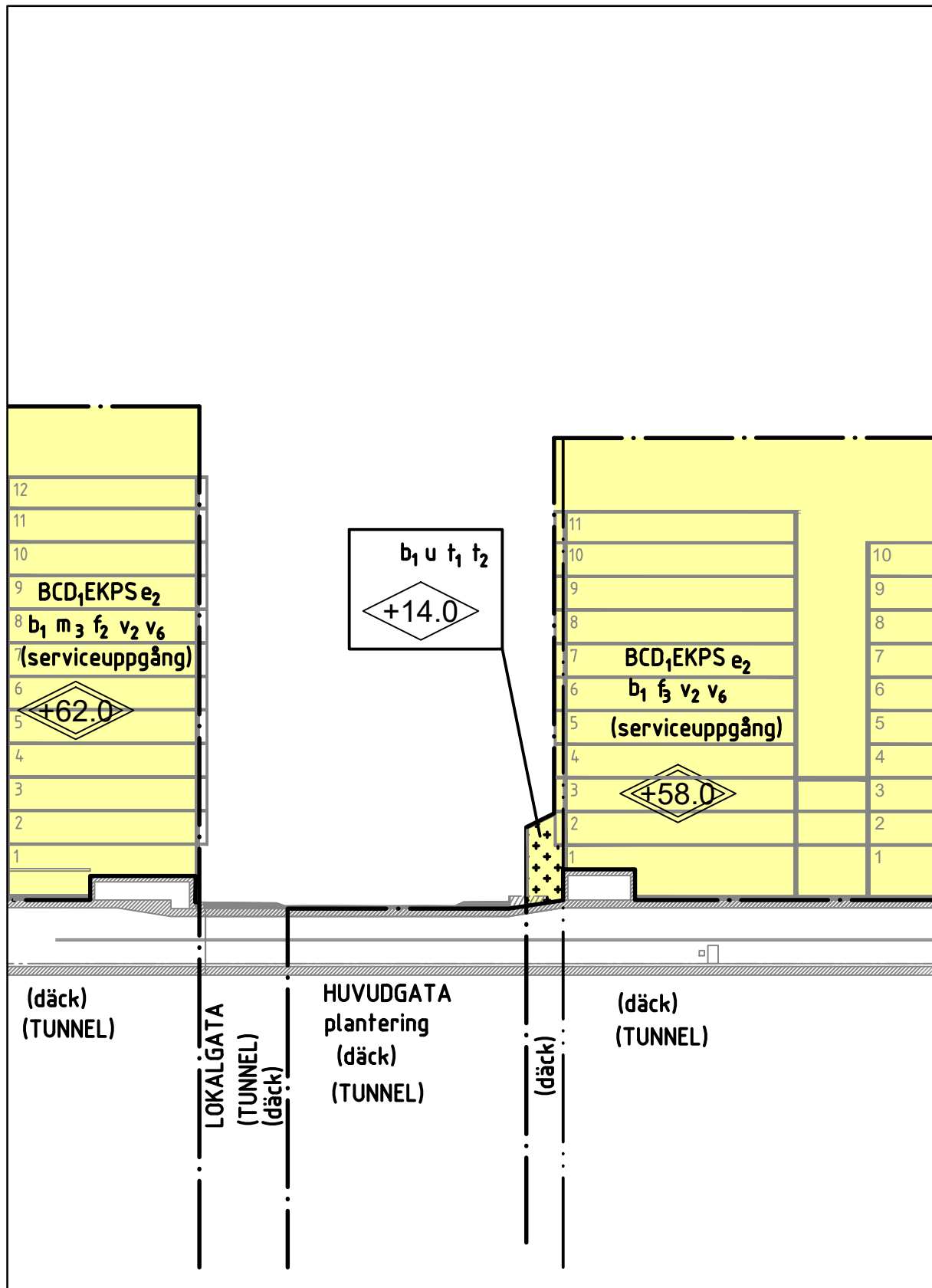
Sektion E-E
