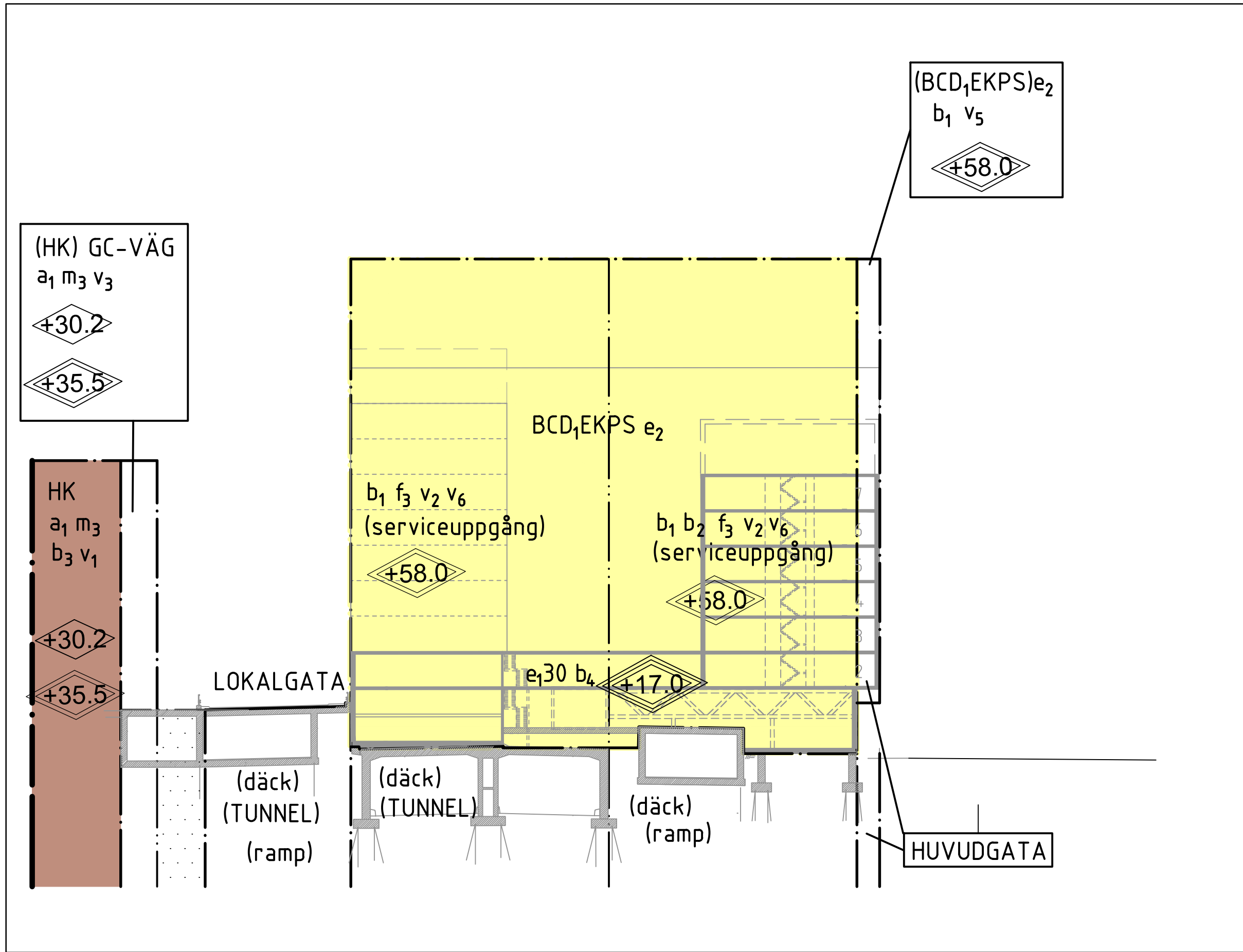
Sektion D-D
