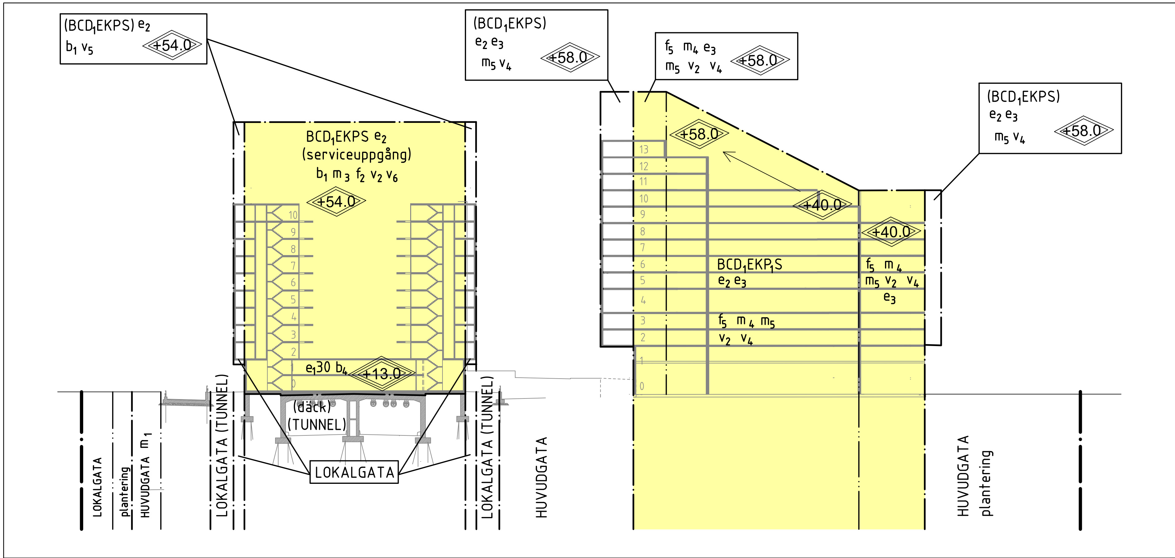
Sektion C-C Sektion genom Kv E går diagonalt genom byggrätten, se sektionlinje på Illustrationsritning 3 av 4
