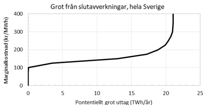
Figur 2. Prognostiserad marginalkostnadskurva för GROT-flis från slutavverkningar
