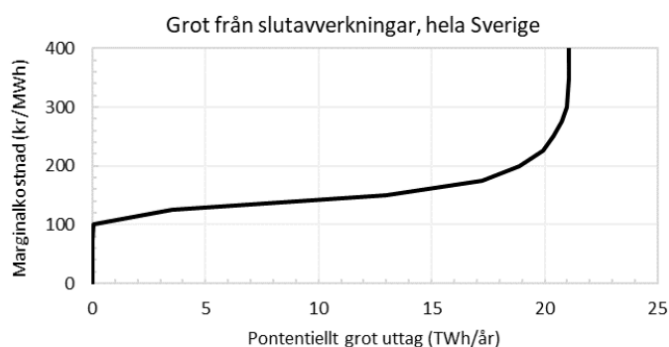
Figur 2. Prognostiserad marginalkostnadskurva för GROT-flis från slutavverkningar
