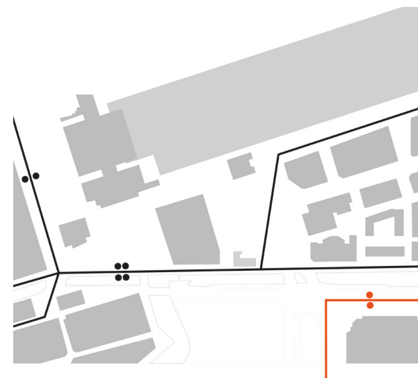
Allélänken etapp 1 och dagens spårlösning vid Åkareplatsen och Drottningtorget
