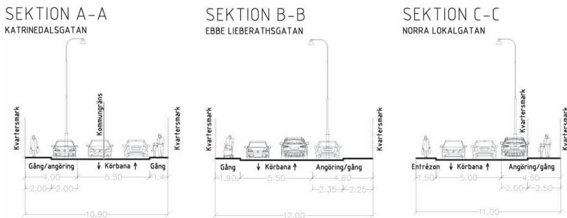
Figur 271: Gatusektioner för omkringliggande gator från trafikförslag (Sweco 2024).
