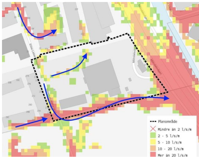
Figur 35: Flöden vid 100-årsregn, nuläge, ur dagvatten- och skyfallsutredningen
