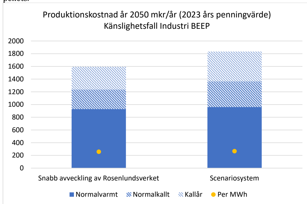
Figur 4: Produktionskostnaderna år 2050 för investeringsalternativen Snabb avveckling av Rosenlundsverket och Scenarioinvesteringar
