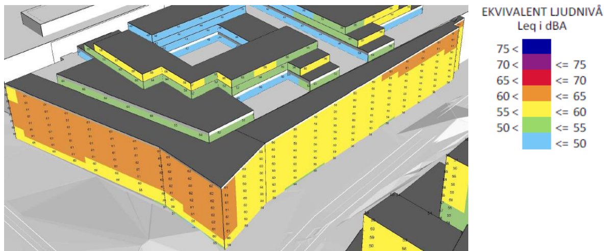
Figur 5-22. Utbyggnad av Nordstan – Det finns goda möjligheter att skapa vanliga bostäder där ljudnivån understiger 60 dBA ekvivalent ljudnivå samt bostäder med en bostadsyta <35 m 2 för fasader i intervallet 60-65 dBA.
