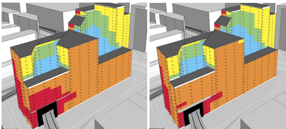
Figur 5-20. Kvarter B-C - Riktvärdet 60 dBA ekvivalent ljudnivå överskrids på flera fasader. Mot innergårdarna finns det goda möjligheter att skapa bostäder då ekvivalenta ljudnivåer förutom för de högsta våningsplanen innehåller 60 dBA. Med införande av en 3 m horisontell skärm ovanför den södra tunnelmynningen kan fler delytor på den östra fasaden innehålla 65 dBA och därmed göras möjliga för bostäder <35 m 2 (höger bild visar bullernivåer utan skärm och vänster bild resultatet med skärm).
