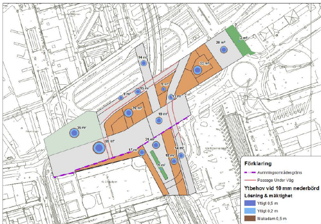
Ytbehov för att fördröja 10 mm nederbörd per hårdgjord yta för de olika delarna inom planområdet, visat för makadam och ytliga magasin med olika mäktighet.
