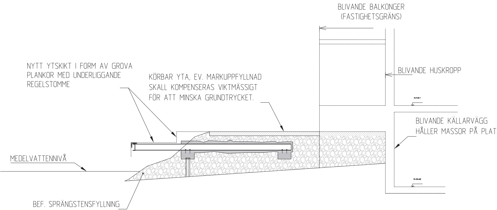
SEKTION A-A SKALA 1:100
