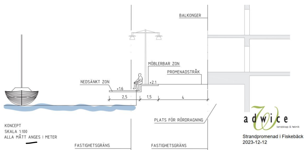
Figur 14. Sektion av strandpromenaden, för detaljer se bilaga 14.
