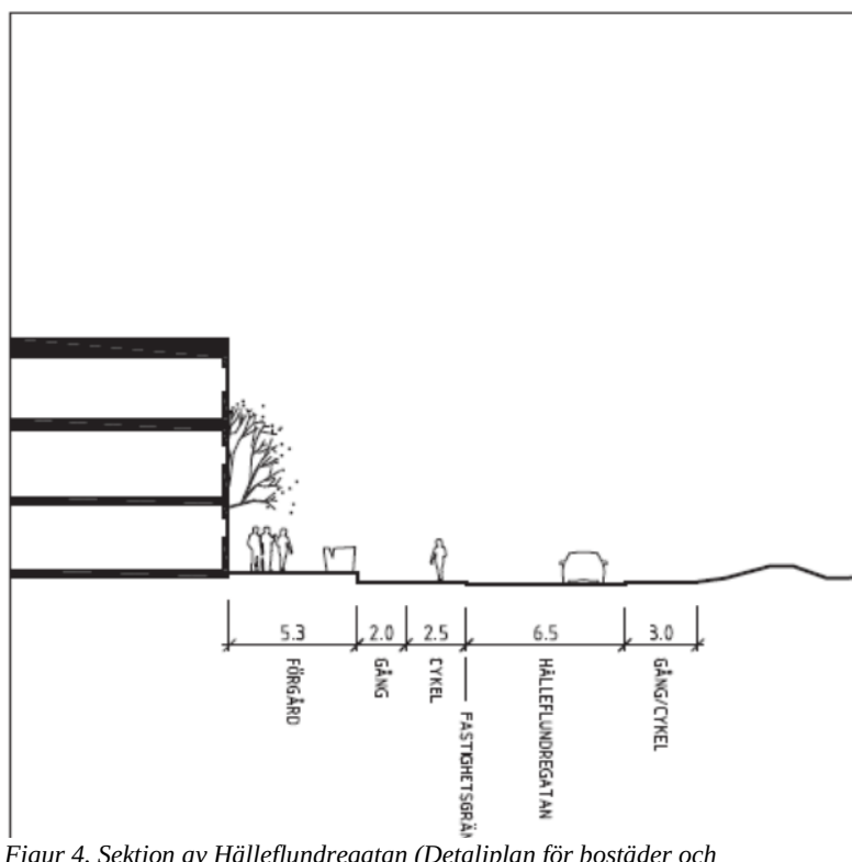
Figur 4. Sektion av Hälleflundregatan (Detaljplan för bostäder och verksamheter vid Hälleflundregatan inom stadsdelen Fiskebäck i Göteborg).
