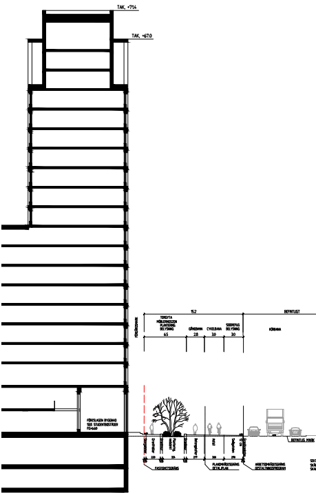
Sektion F-F Skånegatan Skala 1:800 (A4)
