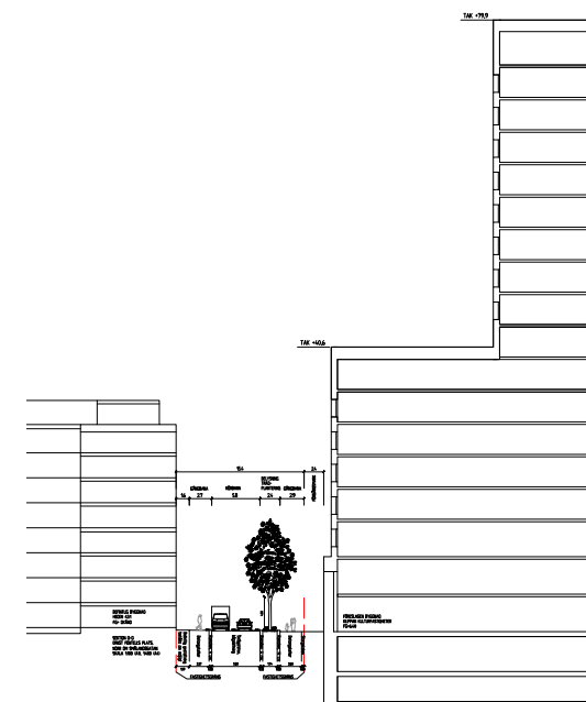
Sektion D-D Ernst Fontells Plats, norr om Smålandsgatan Skala 1:1000 (A4)
