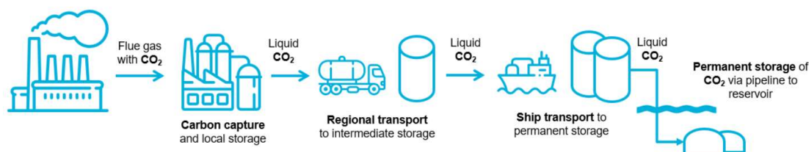
Figur 6. Illustration över hela CCS-kedjan från avskiljning till lagring. Källa Klimakur för avfallsförbrenning i Norge
