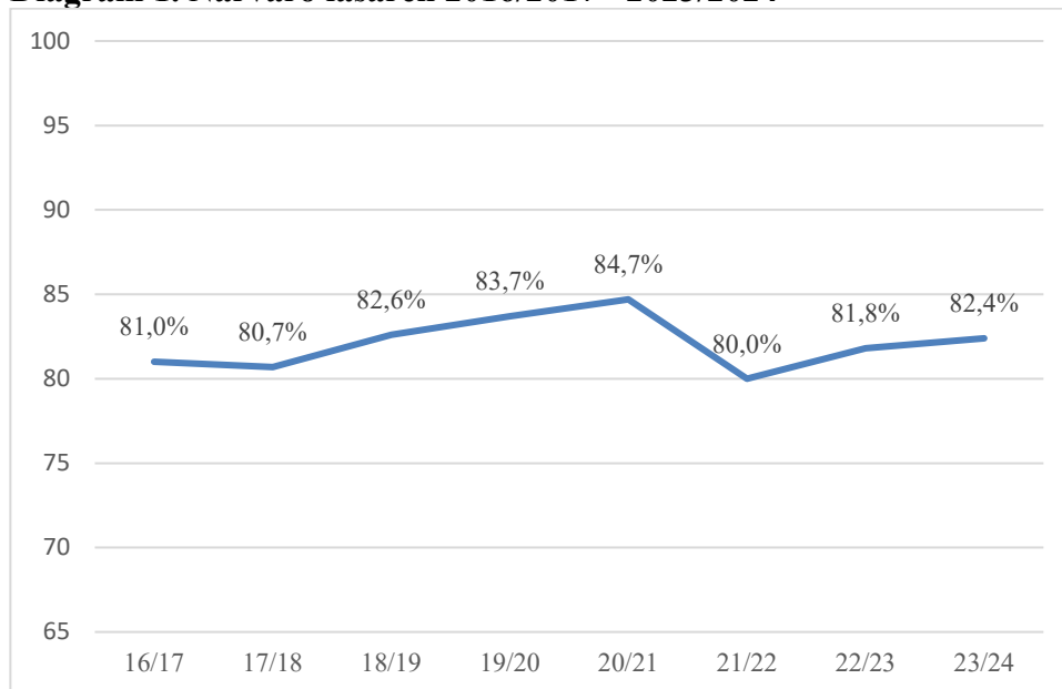
Diagram 1. Närvaro läsår 2016/2017 - 2023/2024
