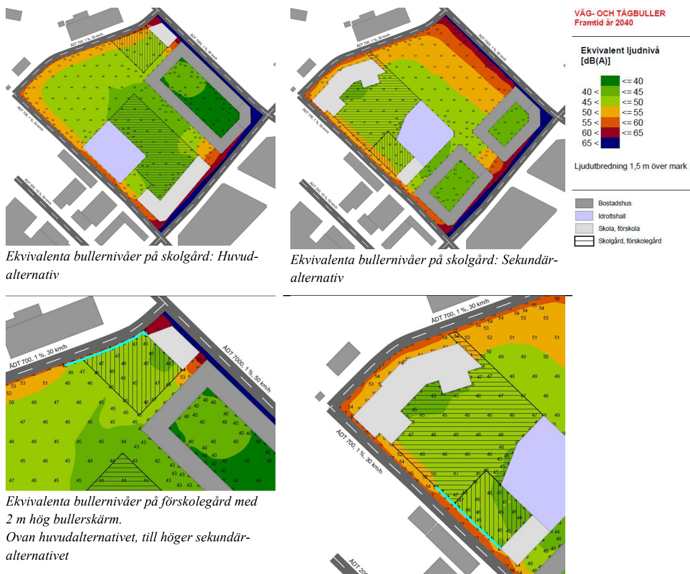
Figur 53. Beräkning av ljudnivå från väg och järnväg på skolgård för två alternativ. Trafikscenariot, bas hög fullt utbyggd 2040 utan åtgärd. (Norconsult 2022-12-14)
