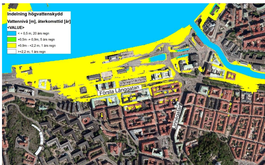
Figur 11. Indelning av högvattenskydd efter återkomsttid och vattennivå inom Linnéstadens avrinningsområde till år 2040.
