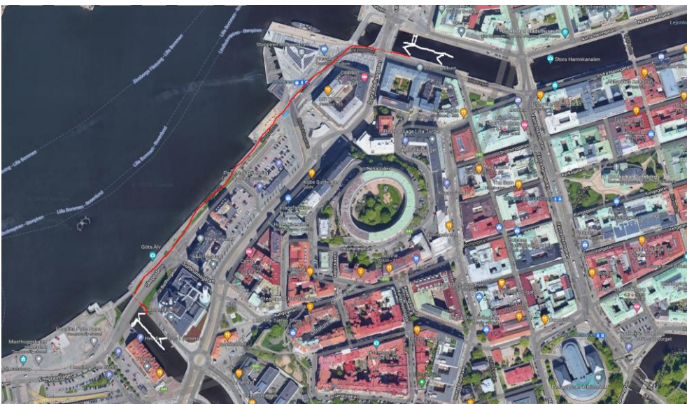
Figur 6. Konceptuell illustration av system med två skydds/slussportar (vitt) samt sträcka för kompletterande inströmningskydd (rött).
