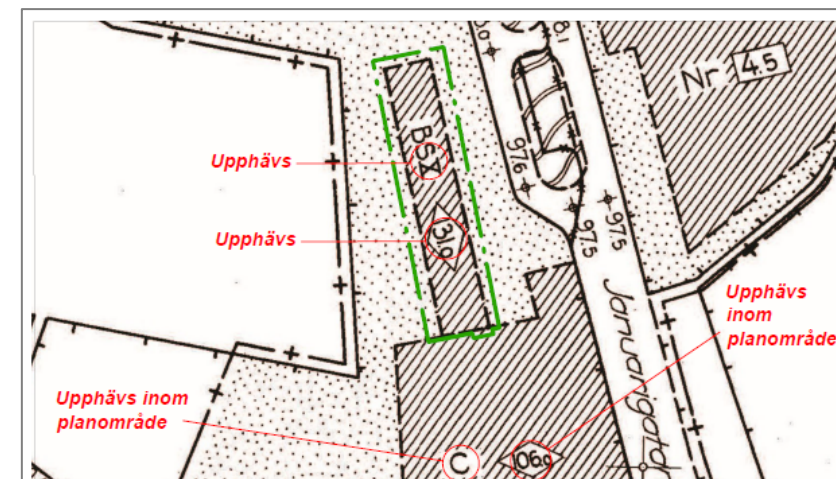
Stadsplan 1480K-II-2789 (ej skalenlig)
