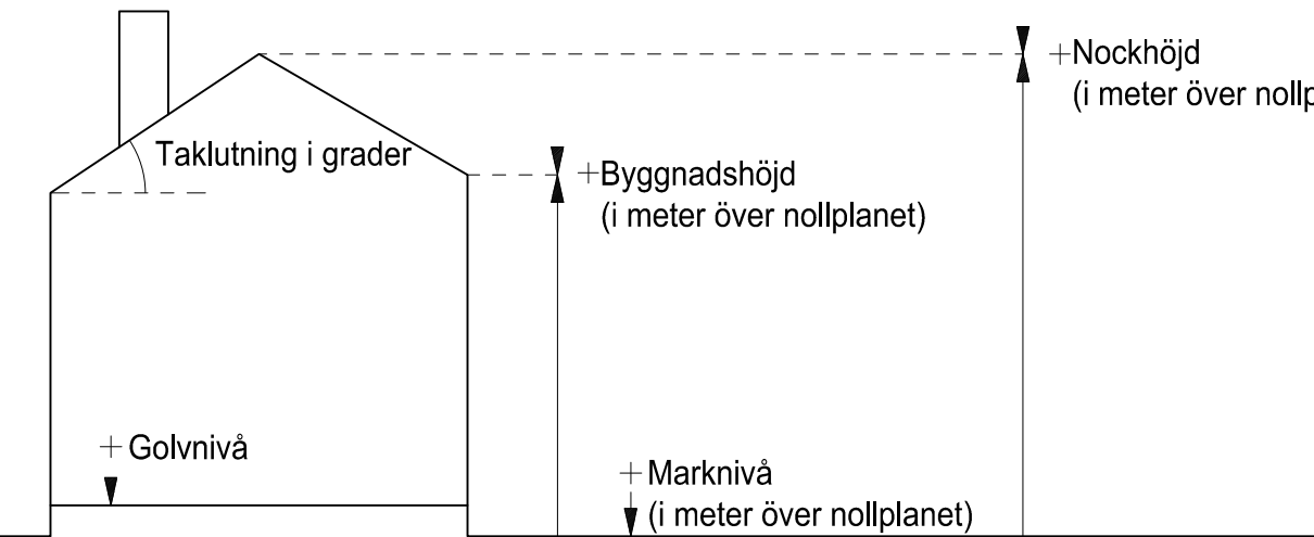
Principskiss över hur höjder och taktutting beräknas
