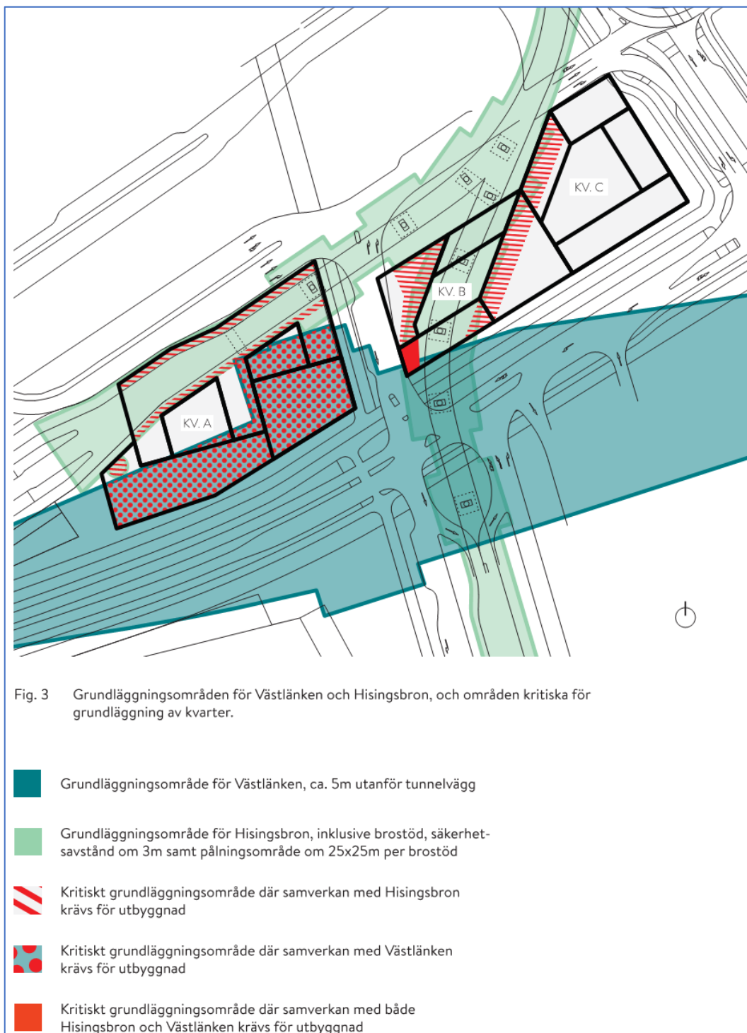
Figur 5-5. Olika byggnadsverks påverkan på varandras grundläggning (Kjällgren Kaminsky & COWI)
