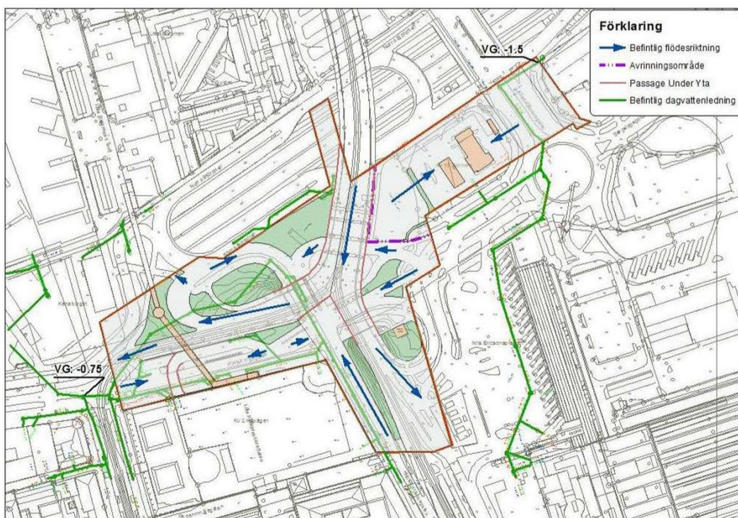
Figur 5-6. Dagvattenflödet i planområdet i nuläget.
