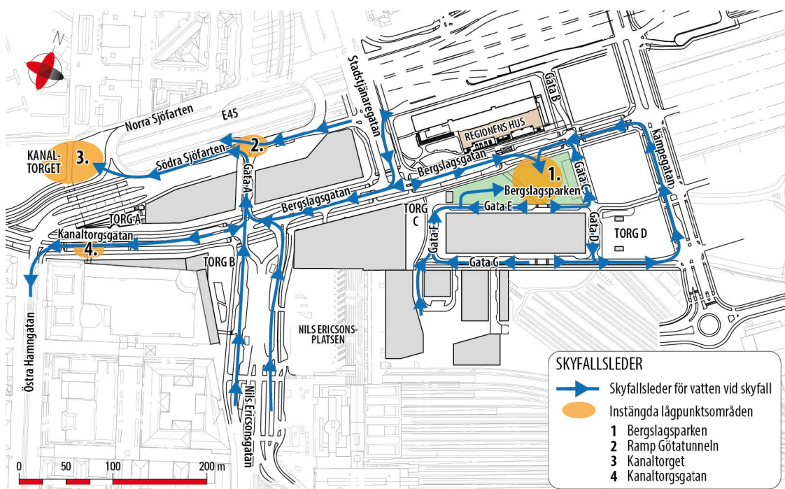
Illustration av skyfallsleder (blå pilar) för vatten vid skyfall samt instängda lågpunktsområden, markerade med orange cirkel numrerade 1-4, inom arbetsområdet
