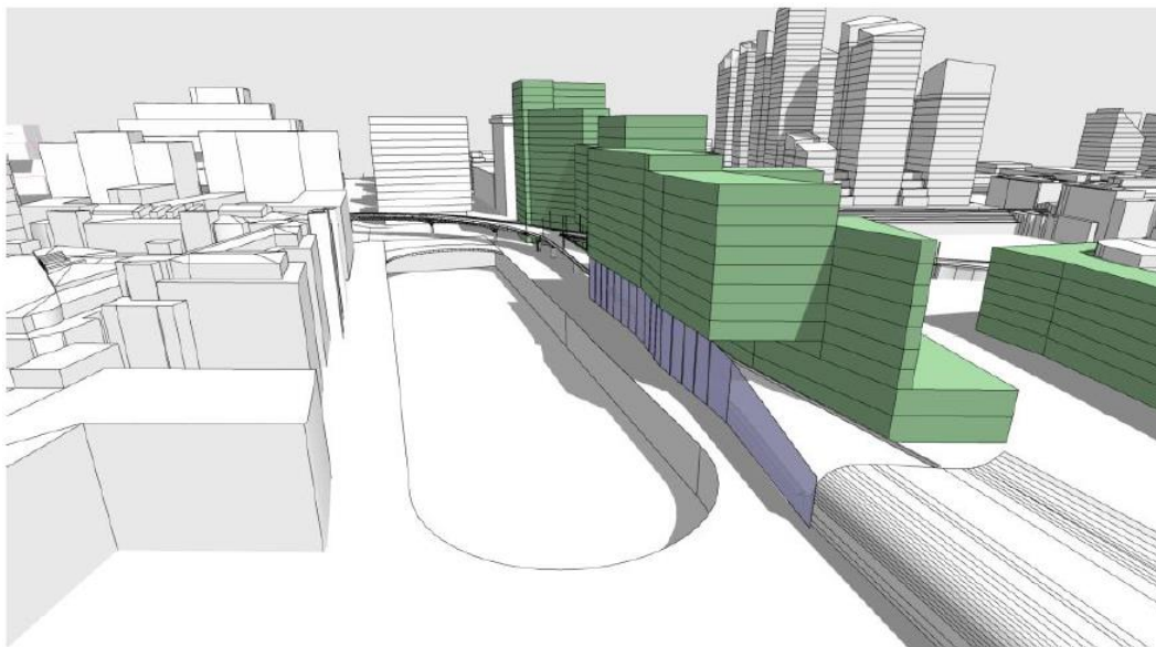
Figur 5-12. Scenario 5 - Förlängd överdäckning och en minst 8 meter hög vägg längs husfasader norr om Nordstan fram till hållplats Kanaltorget (år 2026).
