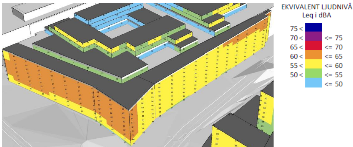
Figur 5-22. Utbyggnad av Nordstan – Det finns goda möjligheter att skapa vanliga bostäder där ljudnivån understiger 60 dBA ekvivalent ljudnivå samt bostäder med en bostadsyta <35 m 2 för fasader i intervallet 60-65 dBA.
