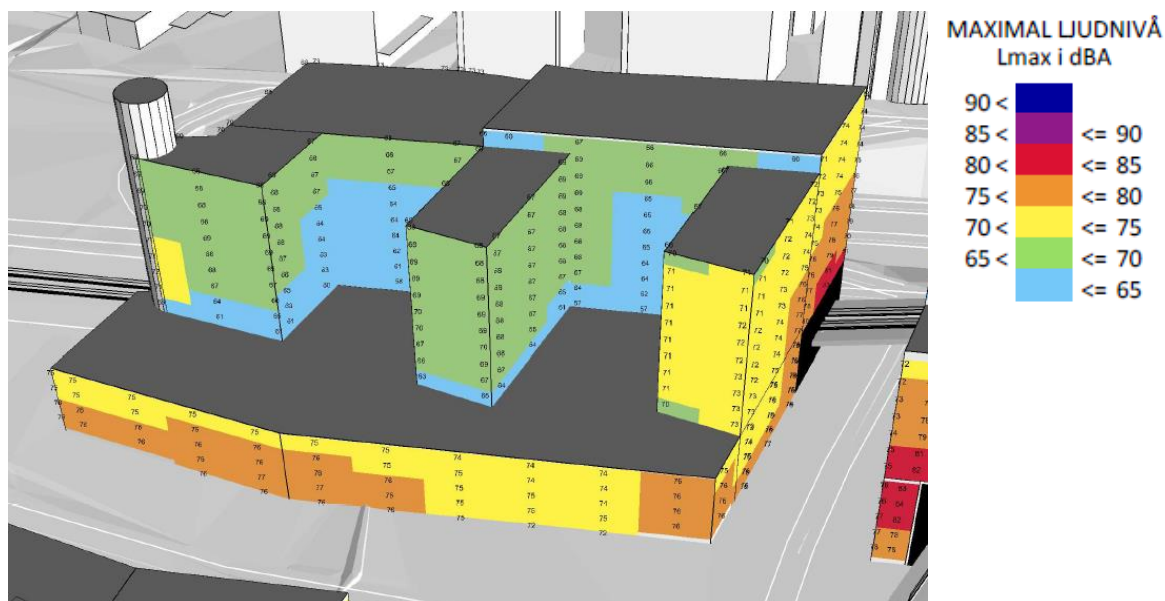
Figur 5-19. Kvarter A - Maximala ljudnivåer överskrider 70 dBA för samtliga fasader utom vissa fasader som vetter mot söder och fasader på innergårdar.
