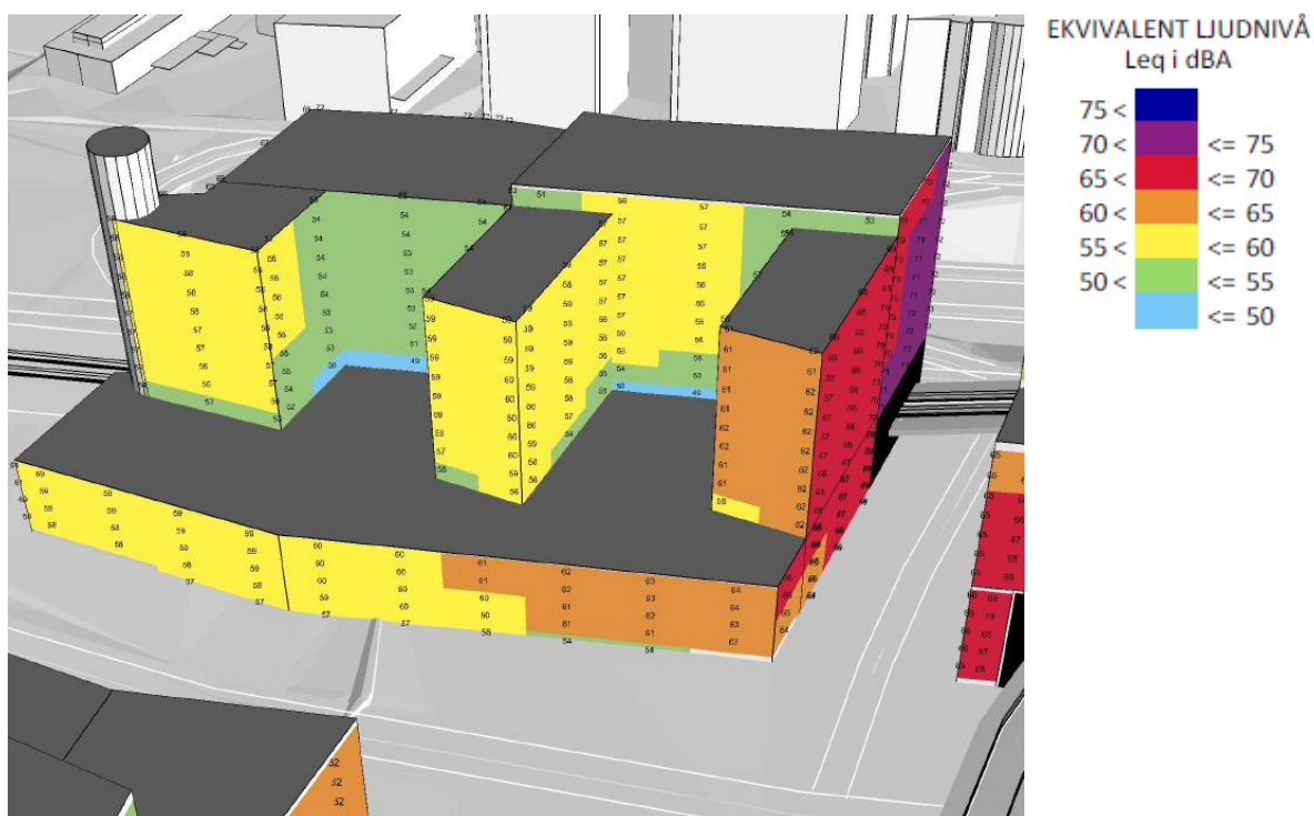
Figur 5-18. Kvarter A - Riktvärdet 60 dBA ekvivalent ljudnivå vid fasad på byggnad A beräknas överskridas på flera fasader. Det finns dock goda möjligheter till bostäder utmed byggnadens södra delar. För delar av byggnaden på den västra och den östra delen av den södra fasaden går det att skapa enkelsidiga bostäder med en bostadsyta <35 m 2 .
