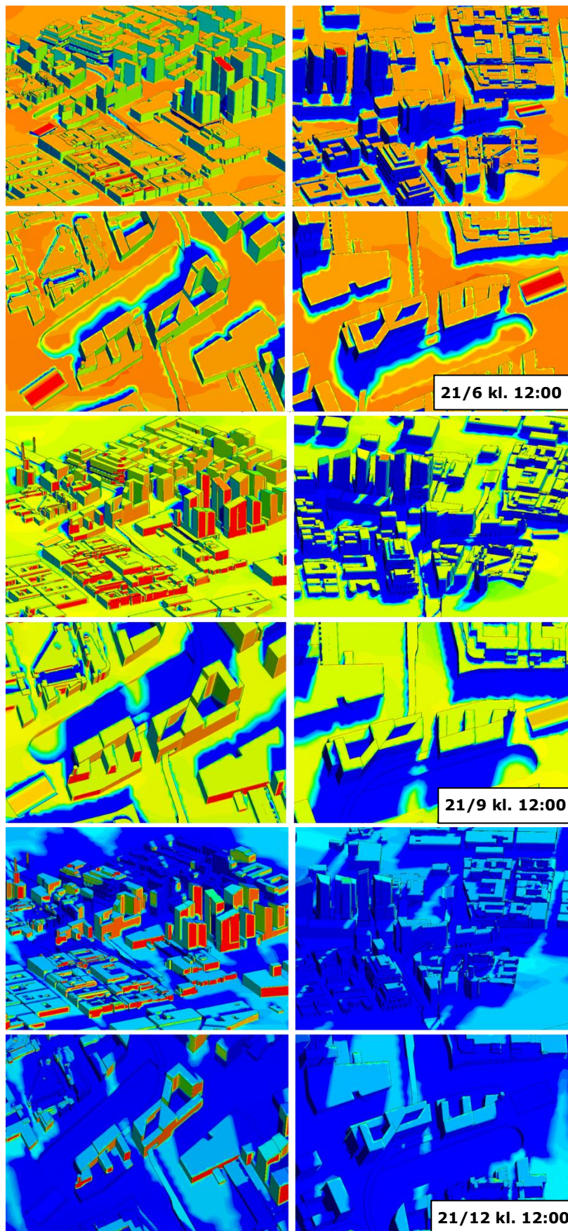
Figur 5-35. Solinstrålning i planområdet för respektive årstid (vår, sommar, höst, vinter).
