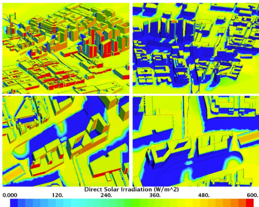
Figur 2 Solinstrålning den 21 juni kl 12. Strålningen är angiven i \text{W/m}^2 .
