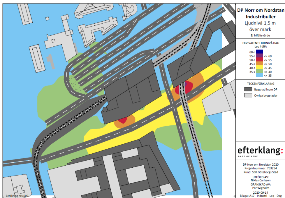
Figur 5-27. Ekvivalenta ljudnivåer för industribuller, dag utomhus 1,5 m över mark.
