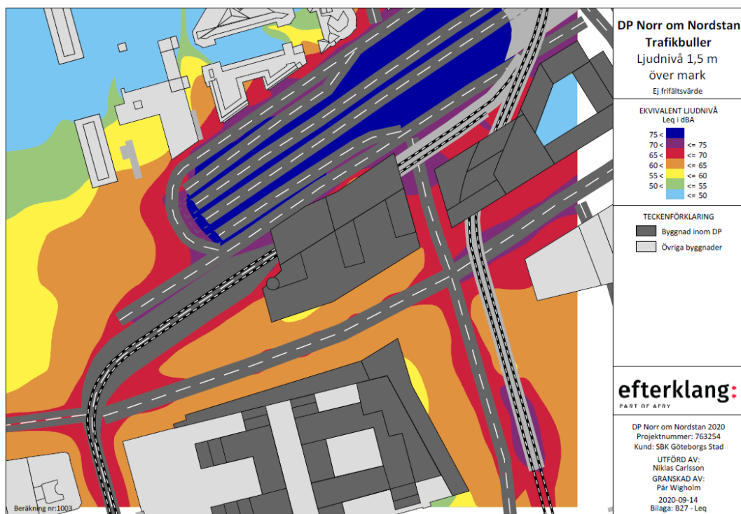
Figur 5-24. Ekvivalenta ljudnivåer för trafikbuller, utomhus 1,5 m över mark.
