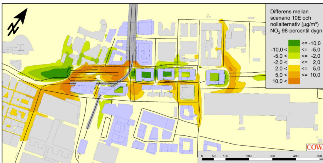
Skillnad i beräknade halter för 98-percentilen av dygnsmedelvärdena av NO 2 , mellan scenario 10E och nollalternativet. Grön skala visar områden där halterna är lägre i scenario 10E, gul/orange skala visar områden där halterna är lägre i nollalternativet.
