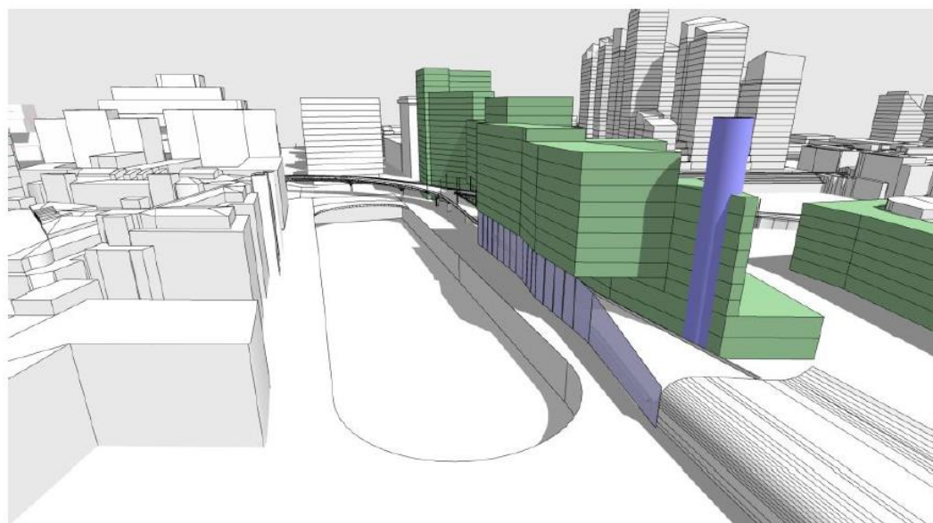
Figur 5-11. Scenario 4 - Samma utformning som i scenario 3 men i scenariot ingår även ett 50 meter högt ventilationstorn som ventilerar bort 95% av emissionerna som sker i Götatunneln. Enbart 5% av emissionerna beräknas i scenariot släppas ut i Götatunnelns mynning (år 2028).
