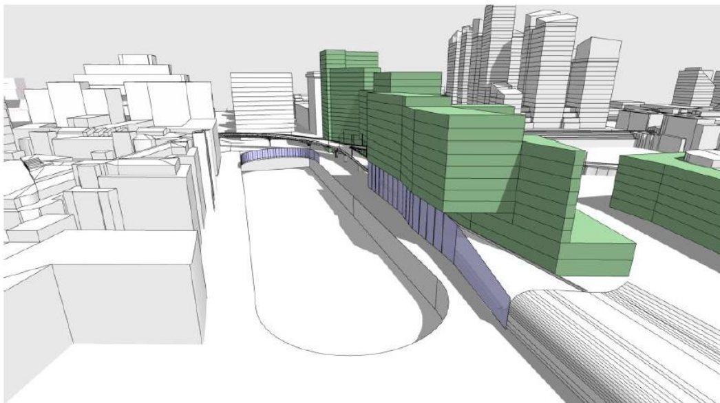
Figur 5-10. Scenario 3 - Förlängd överdäckning, en 6 meter hög skärm på Bananbron vid överdäckningens västra tunnelmynning och en minst 8 meter hög vägg längs husfasader norr om Nordstan fram till hållplats Kanaltorget (år 2028).
