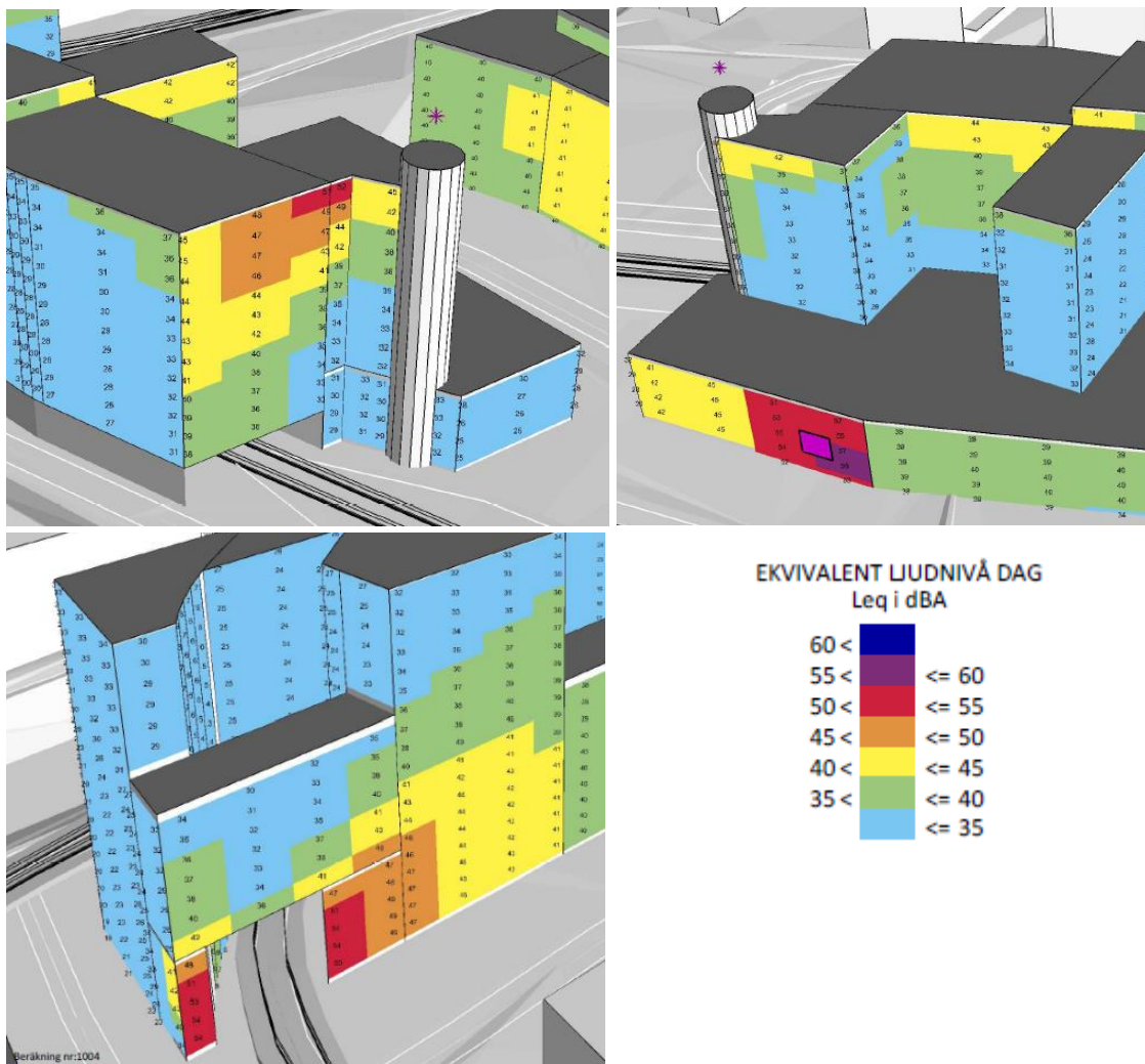
Figur 5-26. Områden på fasader där ljudnivåer överstiger 45 dBA ekvivalent nivå.
