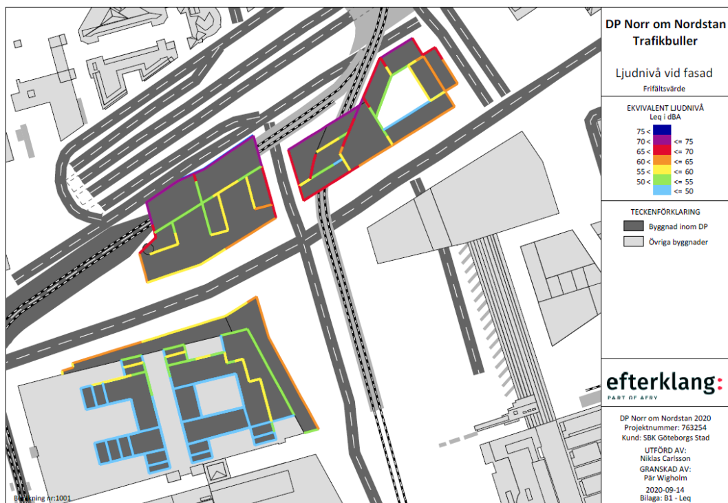
Figur 5-17. Ekvivalent ljudnivå vid fasad, frifältsvärde Leq i dBA
