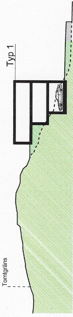
Sektion A-A
