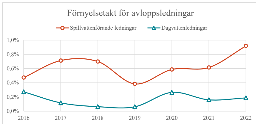
Figur 6 Den historiska förnyelsetakten för spillvattenförande ledningar och dagvattenledningar redovisat för perioden 2016 – 2022.
