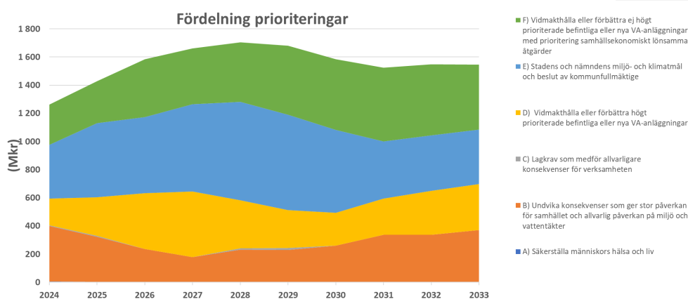
Figur 20 Visuellt exempel på hur alla investeringar och reinvesteringar för vatten och avlopp kan placeras i lämplig prioriteringsgrupp A-F, där grupp A (högst prioriterad) är blått, längst ned.
