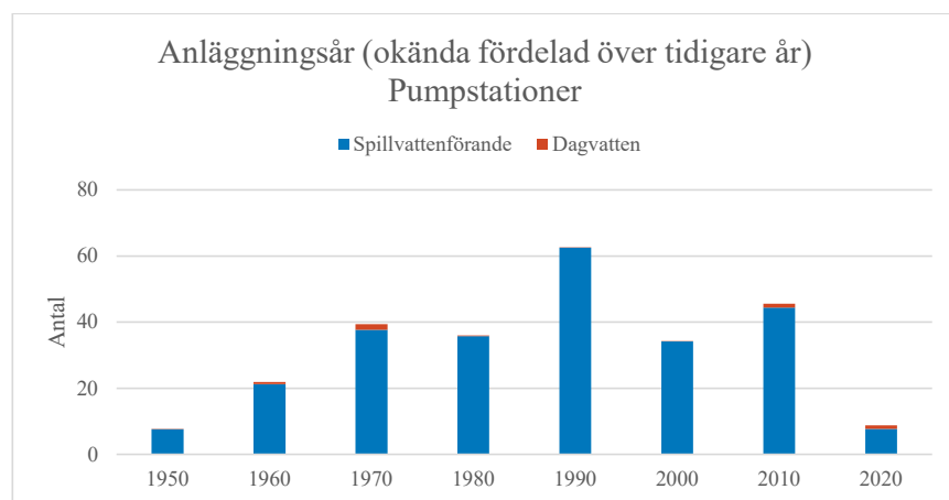
Figur 17 Figur som visar uppskattat anläggningsår för avloppspumpstationer. Notera att för cirka 30 % av stationerna, vilka saknar noterat anläggningsår, har åldern uppskattats baserat på utbyggnadstakten på avloppsledningsnätet.
