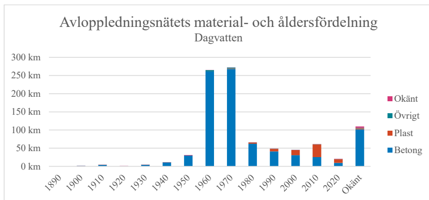
Figur 4 Dagvattenledningsnätets nuvarande material- och åldersfördelning.
