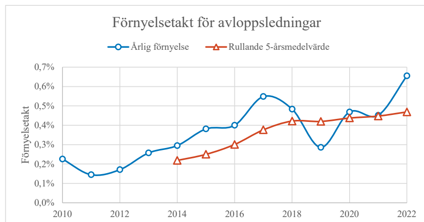
Figur 16 Figur som visar förnyelsetakten på avloppsledningar per år samt som rullande 5-årsmedelvärde.
