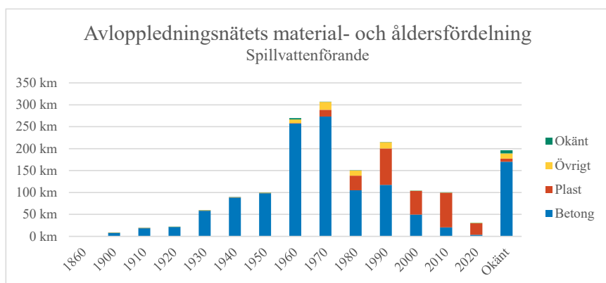
Figur 3 Det spillvattenförande ledningsnätets nuvarande material- och åldersfördelning.
