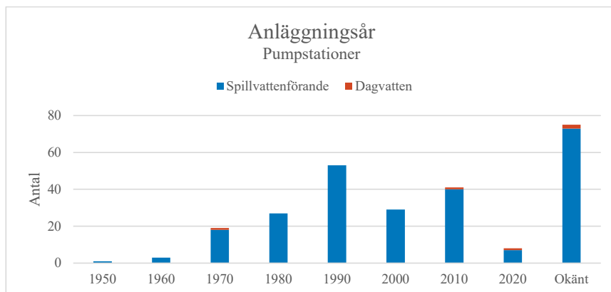
Figur 7 Anläggningsår för avloppspumpstationer.
