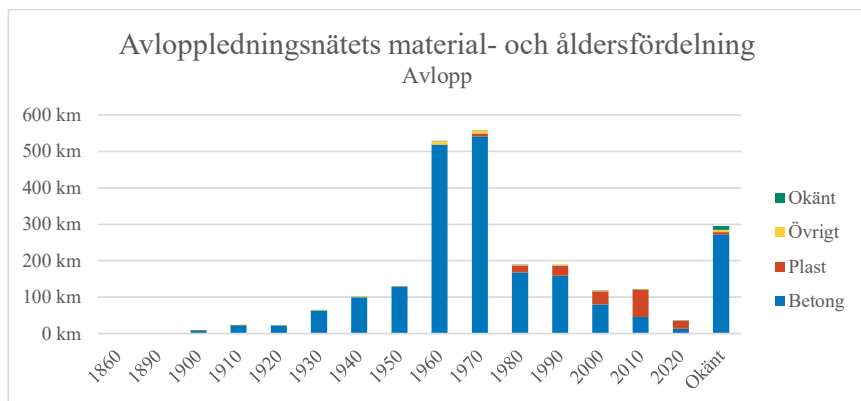
Figur 2 Avloppsledningsnätets nuvarande material- och åldersfördelning.
