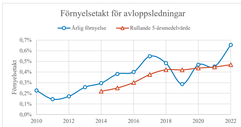
Figur 5 Den historiska förnyelsetakten för avloppsledningar från 2010 fram tills idag.
