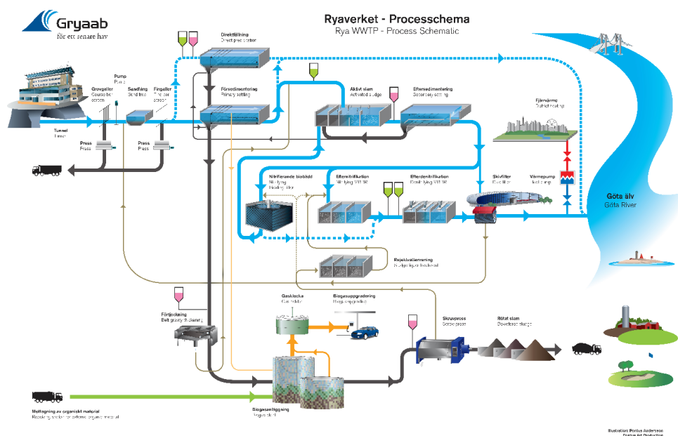
Figur 27 Processchema om flödesvägar genom Ryaverket. Tjocka blåa linjen presenterar huvudflödesvägen av vatten och bruna flödesvägar av slam. Streckade linjen presenterar möjliga vägar för förberedning av flöden.
