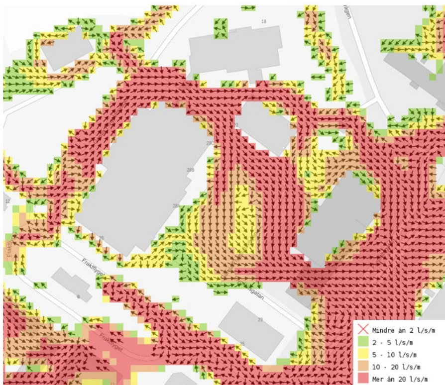
Figur 3, ytvattenflöden inom planområdet vid ett klimatanpassat 100-årsregn.
