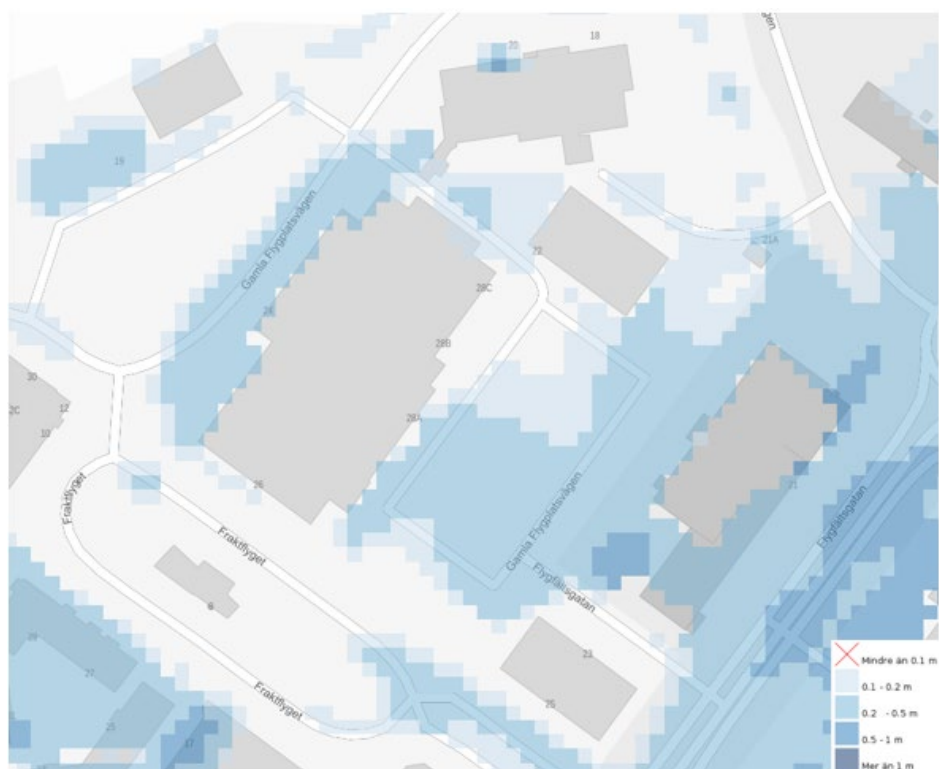
Figur 2, vattennivåer vid ett klimatanpassat 100-årsregn
