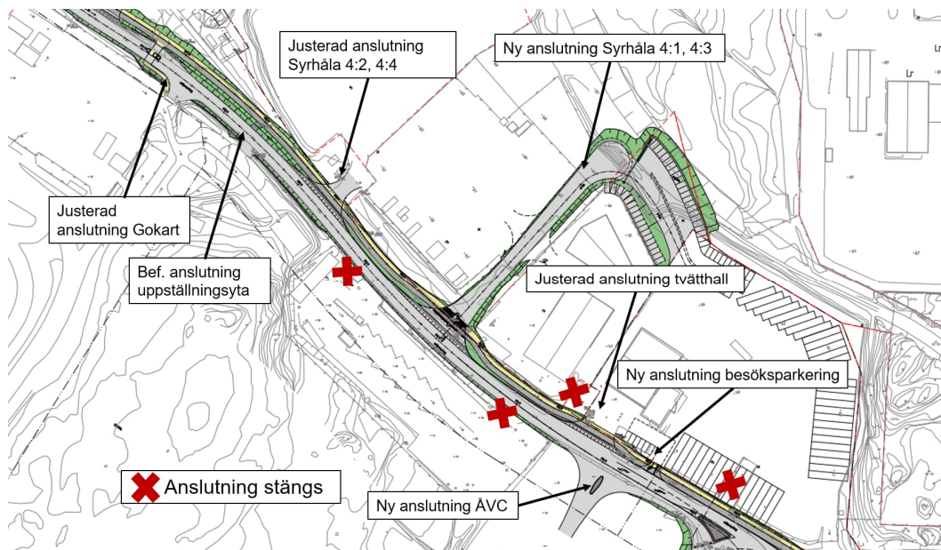
E.1:6 Stängning av anslutningar på sträckan 0/060-0/440.
