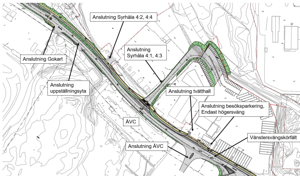
E.1:2 Planutformning 0/060-0/440.
