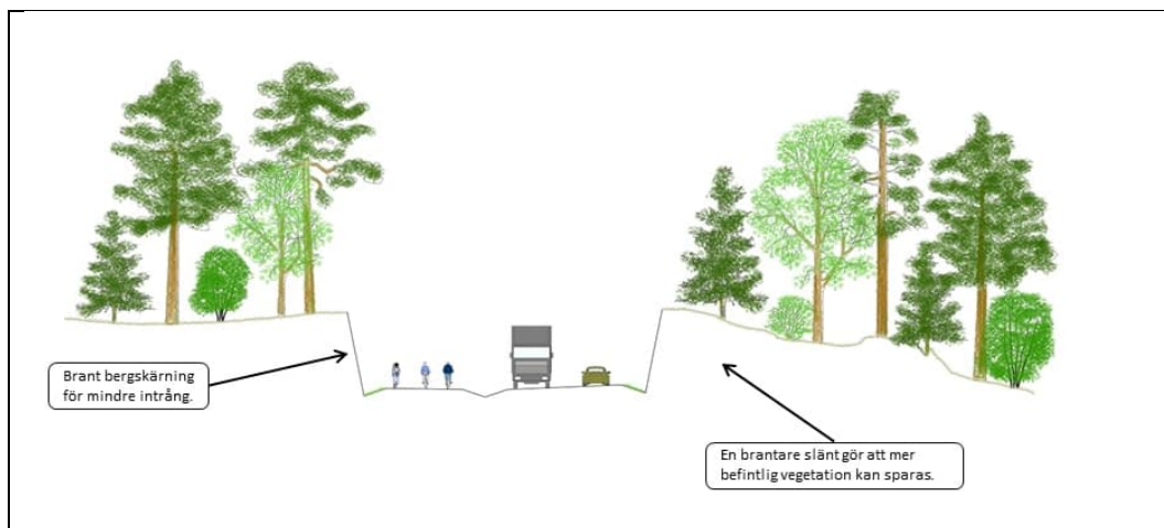
E.1:22 Illustration av sektionsutformning vid dubbelsidig brant skärning, norr om kraftledningsgatan, cirka km 1/500.
