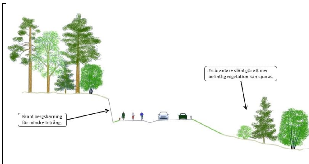
E.1:25 Illustration av sektionsutformning vid enkelsidig skärning och brant yterslänt, söder om kraftledningsgatan, cirka km 1/200.
