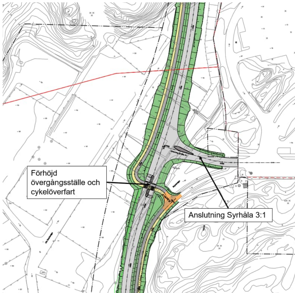
E.1:9 Planutformning 0/900-1/070.
