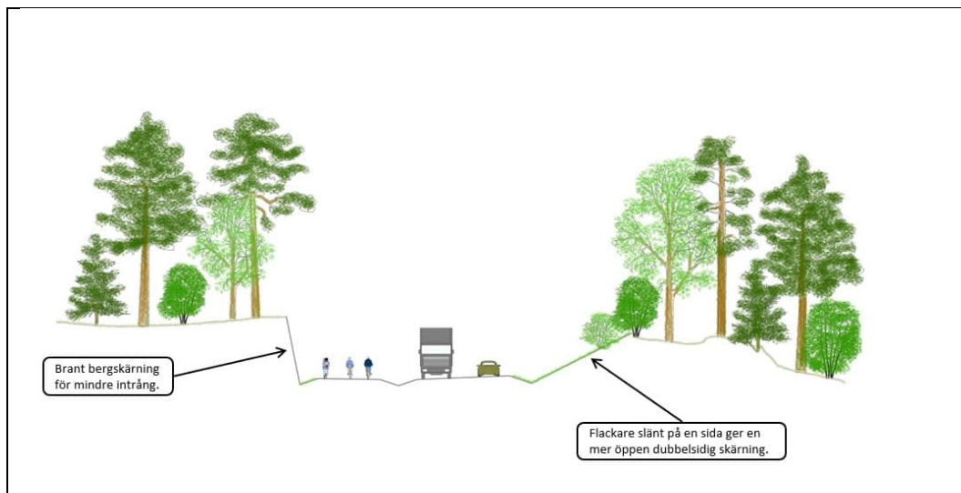
E.1:21 Illustration av sektionsutformning vid dubbelsidig skärning då östra skärningen är flack, norr om kraftledningsgatan, cirka km 1/500.
