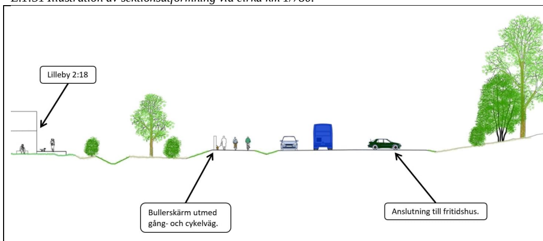
E.1:32 Illustration av sektionutformning vid cirka km 1/800.
