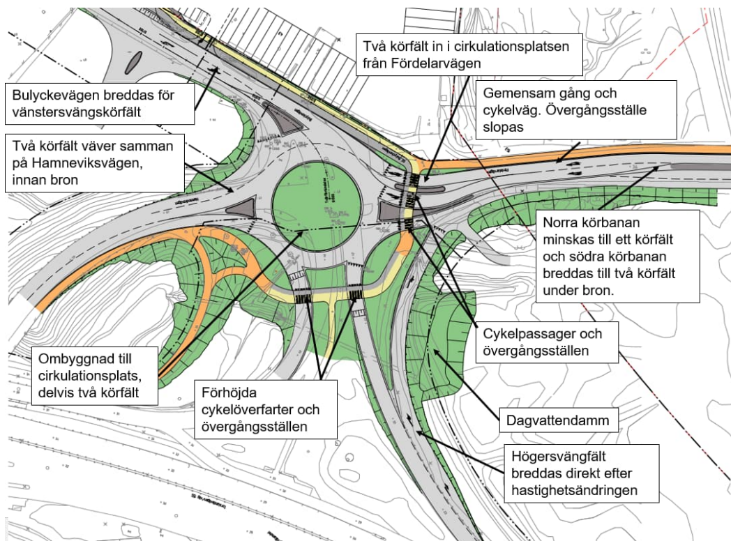
E.1:1 Syrhålamotet, utformningsförslag, delvis tvåfältig cirkulationsplats ersätter signalkorsning.
