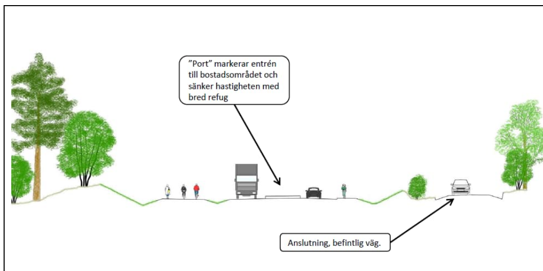
E.1:34 Illustration av sektionsutformning vid "porten" till Älvegårdsområdet, cirka km 2/100.
