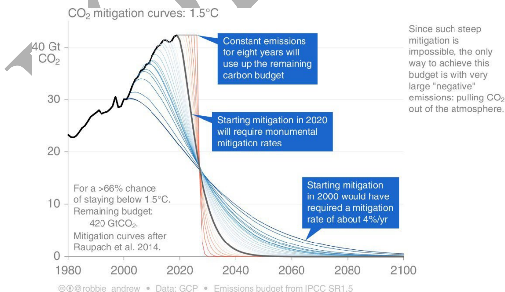
Figur 4. Figuren visar globala utsläppsminskningskurvor som startar vid olika tidpunkter. Samtliga utgår från att begränsa den globala uppvärmningen till 1,5 grad med 66 procent sannolikhet. Detta illustrerar att
