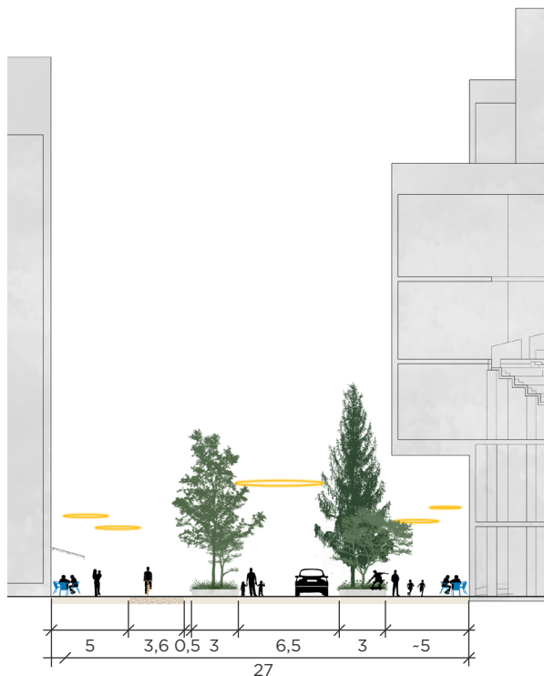
Principsektion för Valhallagatans östra del, mellan arenorna, med 27 meters bredd. Gatan ska gestaltas som ett lågfartsområde där gångytor är prioriterade. Utformningen möjliggör ett flexibelt samnyttjande.
