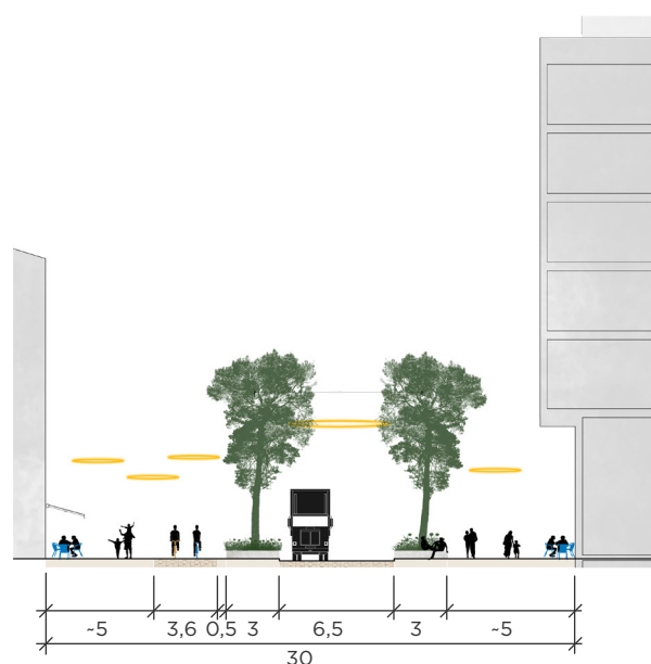
Principsektion för Valhallagatans västra del. Utformningen är mer strikt, med tydlig separering av trafikslagen.
