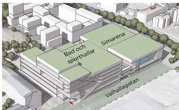
Modellbild. Centralbad, simarena och sporthallar. Röd pil markerar entré från Valhallagatan. Illustration: Norconsult.
