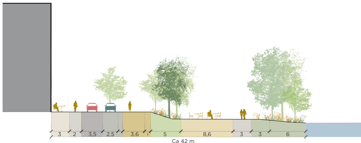
Principsektion A-A för ytan mellan bebyggelsen och å-rummet. Illustration: O2 landskap.
