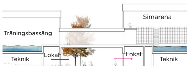
Sektion som visar hur badet sammanlänkas med en passage över den nordsydliga lokalgatan. Illustration: Norconsult.
