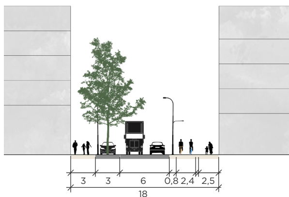
Principsektion för den nya lokalgatan. Illustration: Cowi.
