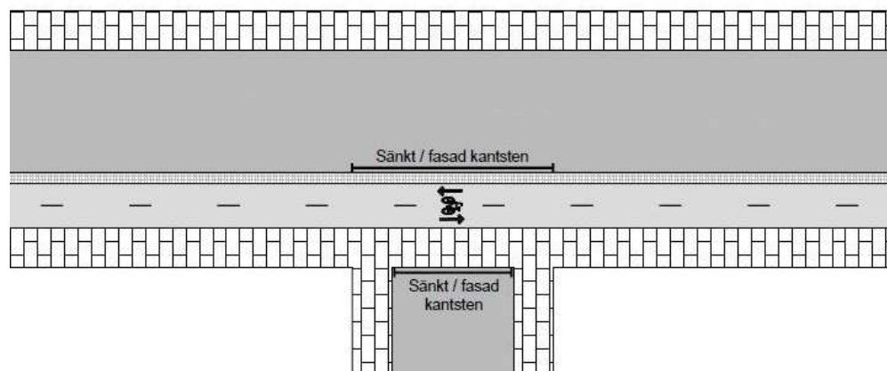
Figur 44. Principiell utformning av genomgående gång- och cykelbana enligt Teknisk Handbok.
