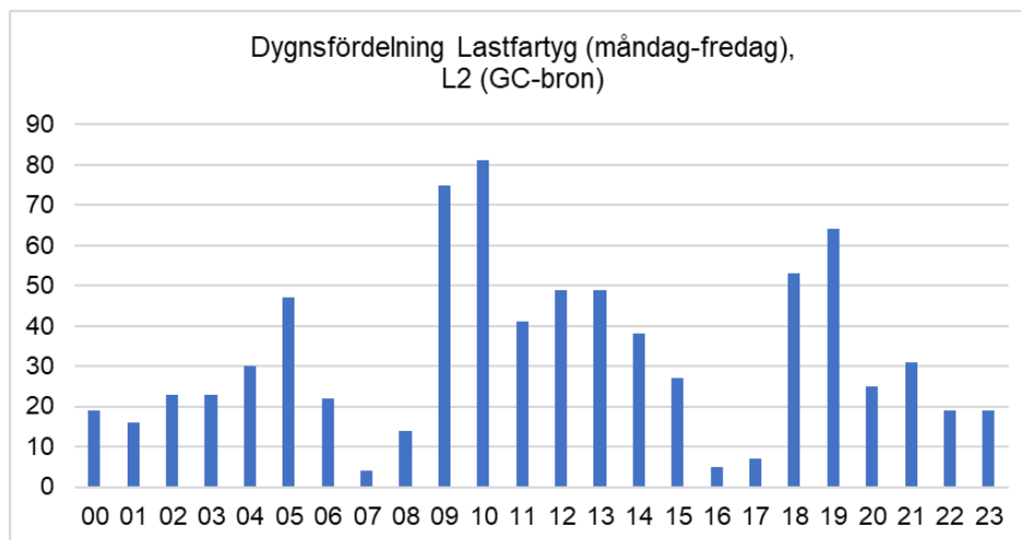
Figur 4:32. Diagram visande passager för fartygskategorin Lastfartyg över passagelinje L2 över dygnet 2023 med lördagar och söndagar bortfiltrerade. Notera att spärrtider förekommer helgfria vardagar mellan klockan 06.00-09.00 och klockan 15.00-18.00.
