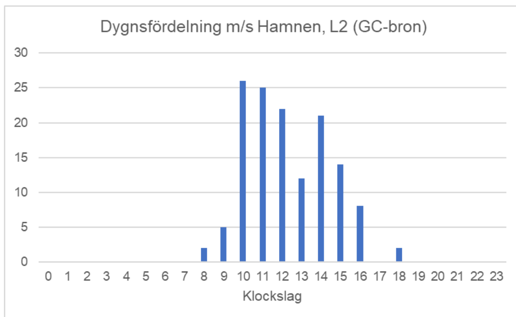
Figur 4:42. Diagram med antal passager för fartyget m/s Hamnen genom läget för planerad gång- och cykelbro under 2023 redovisat över dygnet.
