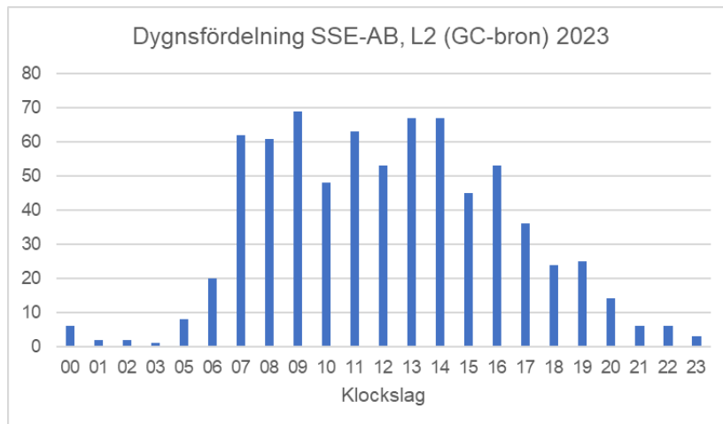
Figur 4:45. Diagram med totalt antal årliga passager fördelade över dygnet för SSE-AB:s fartyg genom läget för planerad gång- och cykelbro under 2023.
