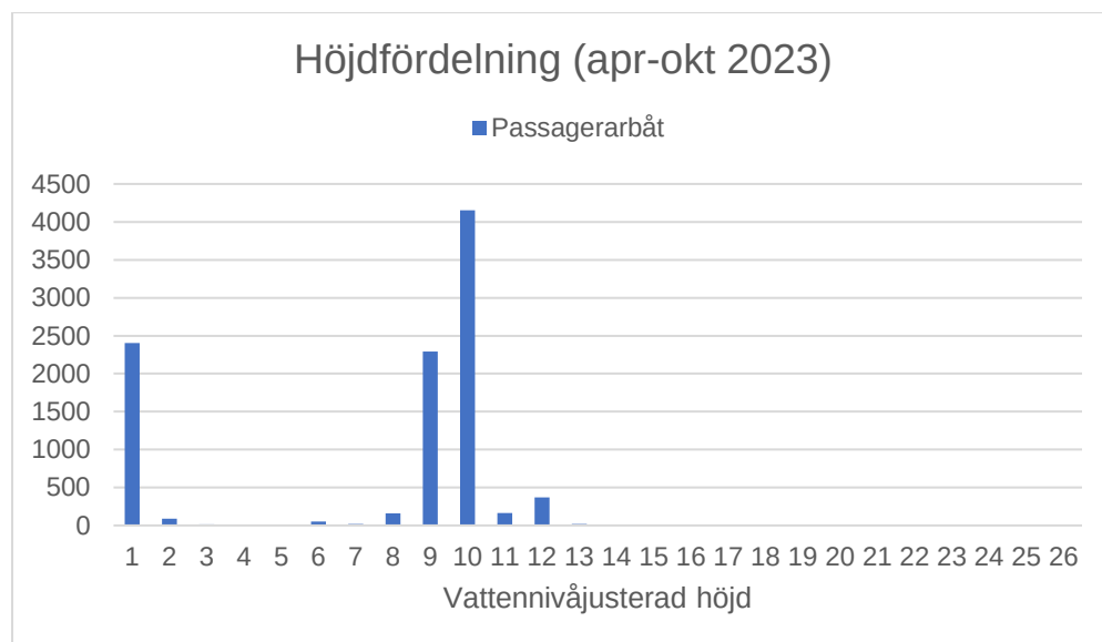
Figur 4:39. Histogram som visar höjdfördelningen av passagerarfartygen i olika höjdistervall. De två vänstra staplarna består uteslutande av Paddanbåtarna och de högra utgör resterande passagerarfartyg.
