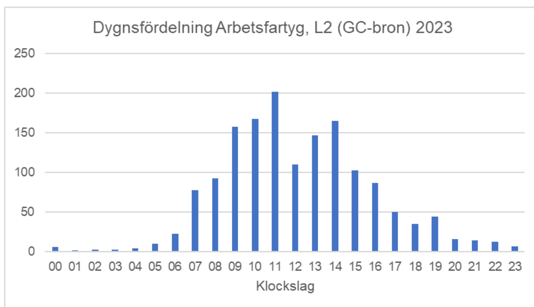
Figur 4:41. Diagram med antal passager fördelade över dygnet för arbetsfartyg genom läget för planerad gång- och cykelbro under 2022.
