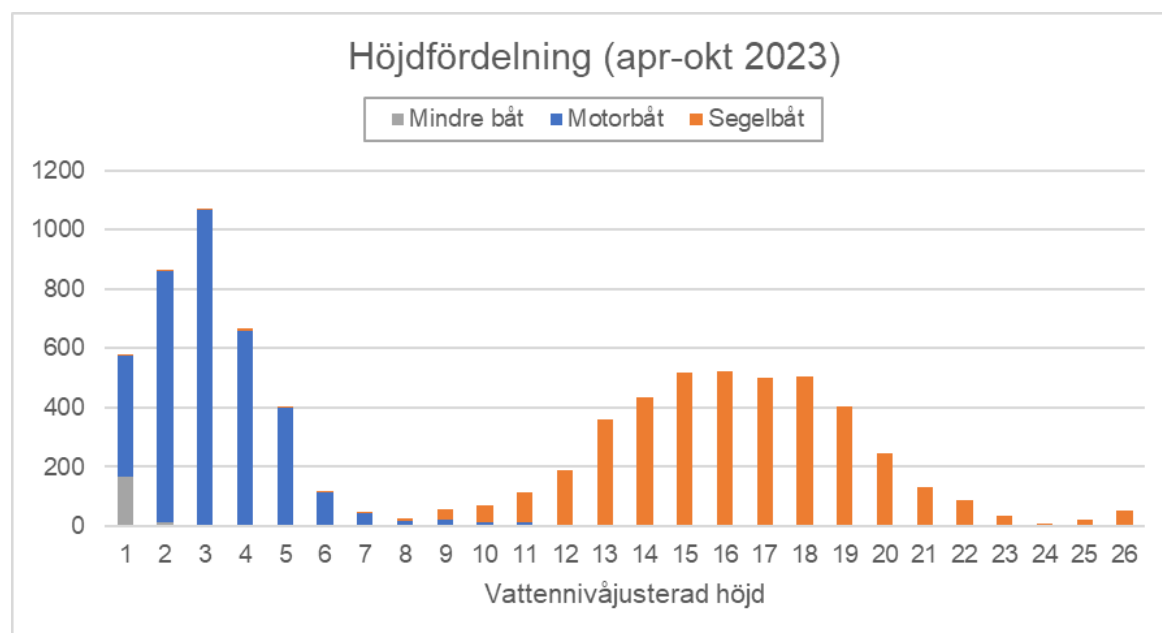
Figur 4:51. Histogram över höjdfördelningar för fritidsfartygen uppdelade på motorbåtar och segelbåtar. Kategorin Mindre båt utgörs av exempelvis kajaker och vattenskotrar.
