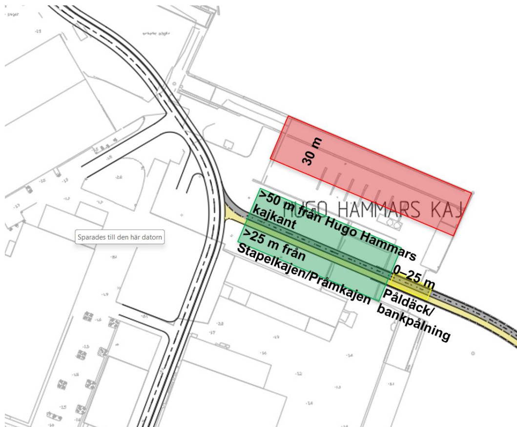
Figur 22 Områdesmarkeringar i plan med olika behov av geoteknisk förstärkning. Inom den övre (röd) områdesmarkering bör gång- och cykelvägen inte placeras på grund av eventuell påverkan på befintlig kaj. Inom den högra nedre (gul) områdesmarkeringen erfordras stabilitetshöjande åtgärder i form av påldäck/bankpållning. Inom den vänstra nedre (grön) områdesmarkering kan gång- och cykelvägen placeras utan geoteknisk förstärkning med hänsyn till stabilitetsförhållandena.
