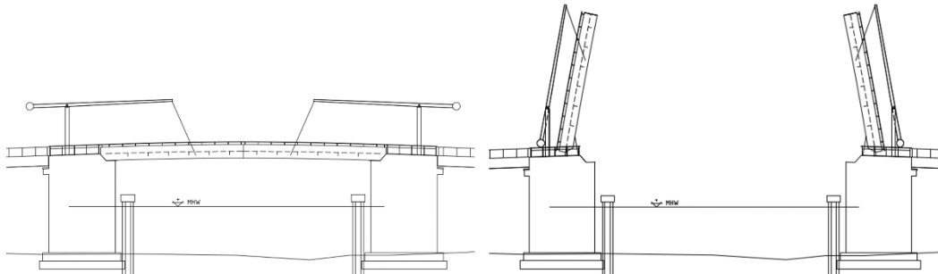
Figur 53 Visar schematisk ett exempel på en dubbelklaffbro med överliggande motvikter.
