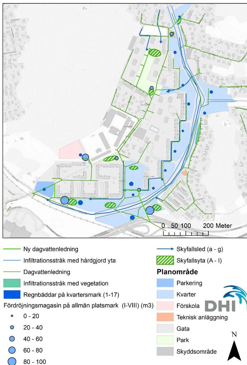
Figur 10 Rekommenderade dagvatten- och skyfallsanläggningar inom planområdet.
