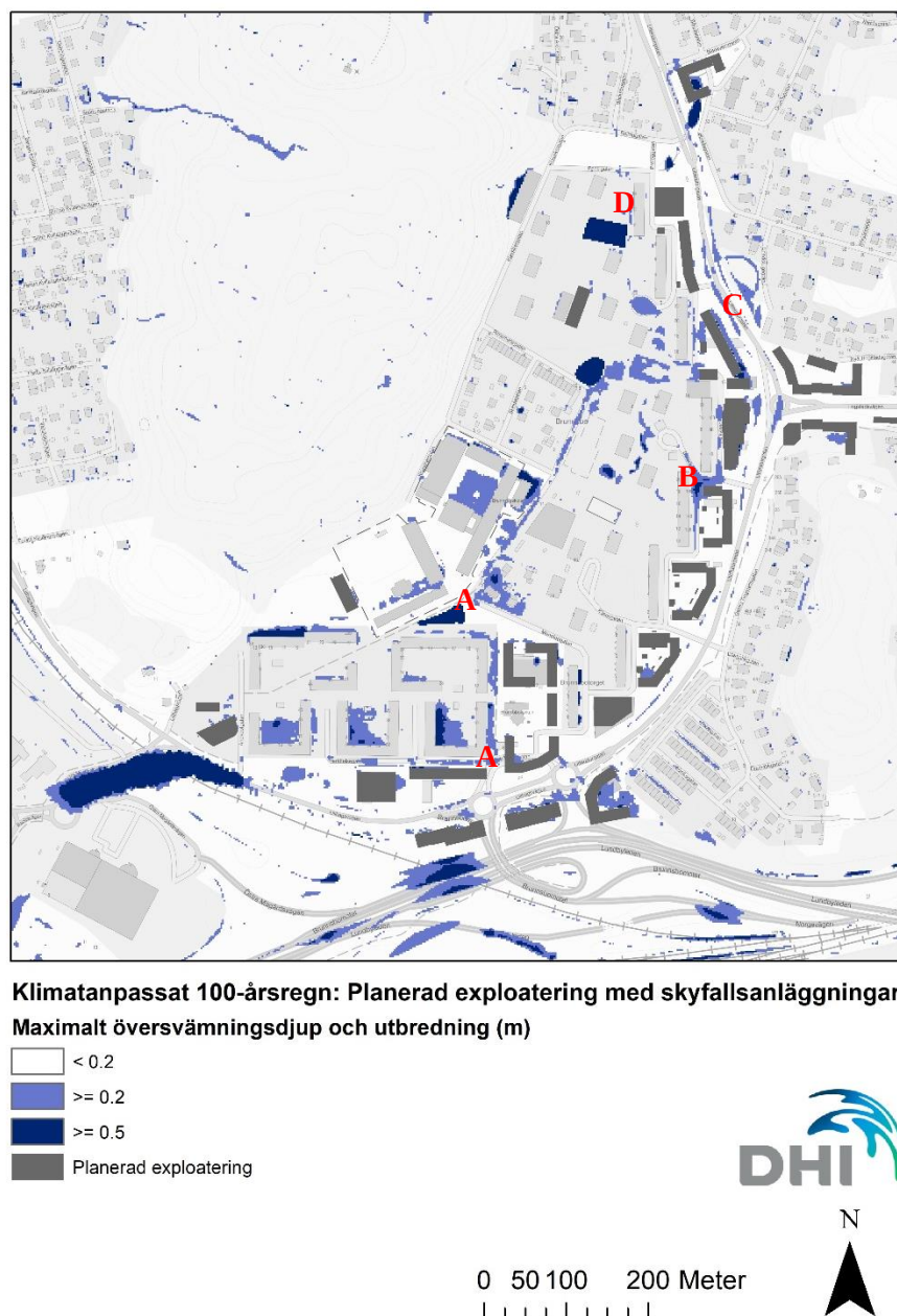
Figur 22 Maximalt översvämningsdjup vid klimatanpassat 100-årsregn för vattennivåer från 20 respektive 50 cm.
