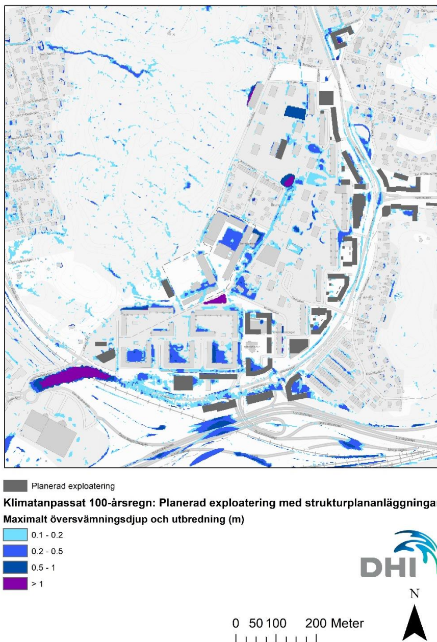
Figur 28 Maximalt översvämningsdjup vid planerad exploatering med rekommenderade skyfallsanläggningar och kompletterande strukturplansanläggningar I och IV presenterade i Figur 11.
