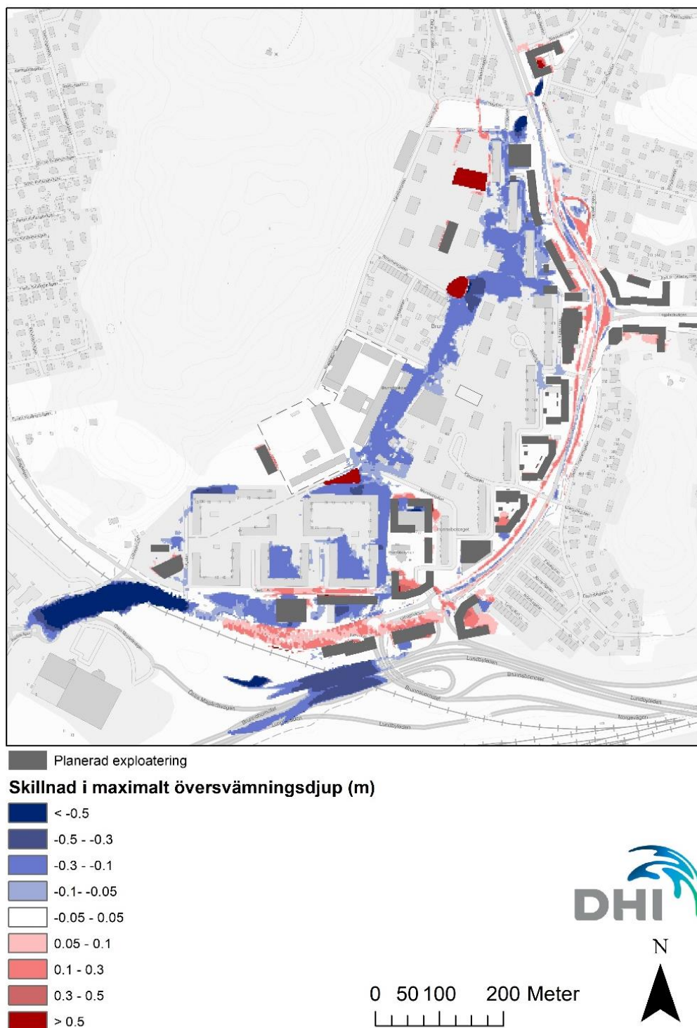
Figur 9 Skillnad i maximalt översvämningsdjup jämfört med nuläge.
