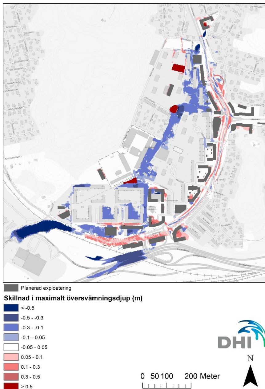
Figur 29 Skillnad i maximalt översvämningsdjup jämfört med nuläge.
