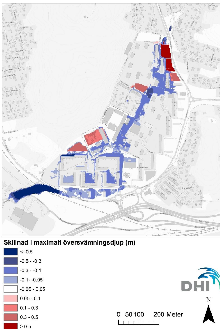
Figur 13 Skillnad i översvämningsdjup (m).
