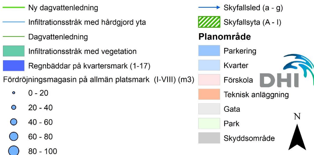
Figur 11 Rekommenderade dagvatten- och skyfallsanläggningar inom norra delen av planområdet.
